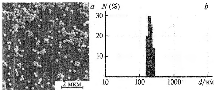
Микрофотографии (a) и гистограммы распределения по размерам (b) частиц полистирольных суспензий, полученных при объемном соотношении стирол/водный раствор F-127, равном 1 : 6, и концентрации, равной 1 мас.% в расчете на мономер.
